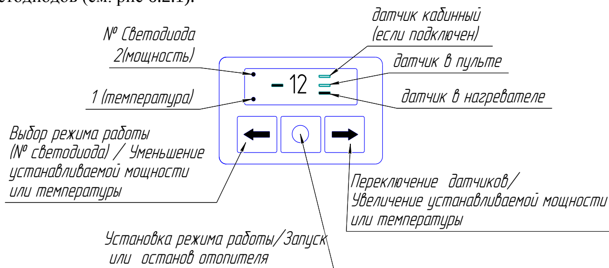
Рис. 6.2.1- Панель пульта
