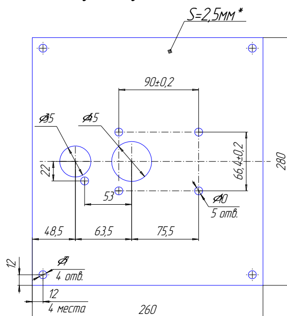
Рис 8.3- Пластина монтажная
