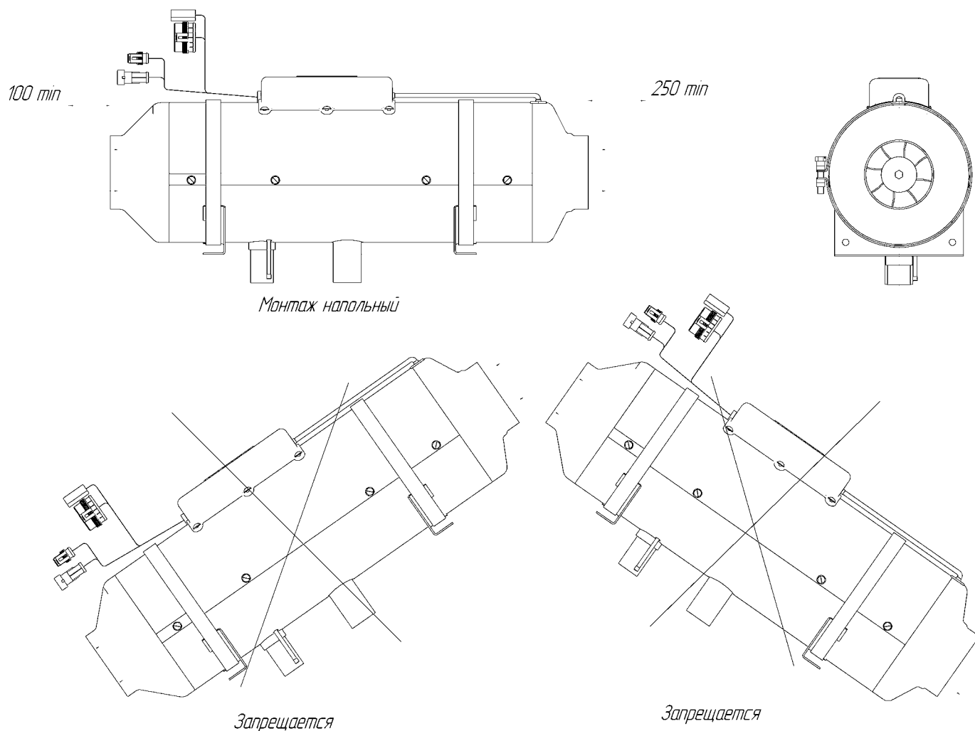
Рис.8.1 – Установка нагревателя
