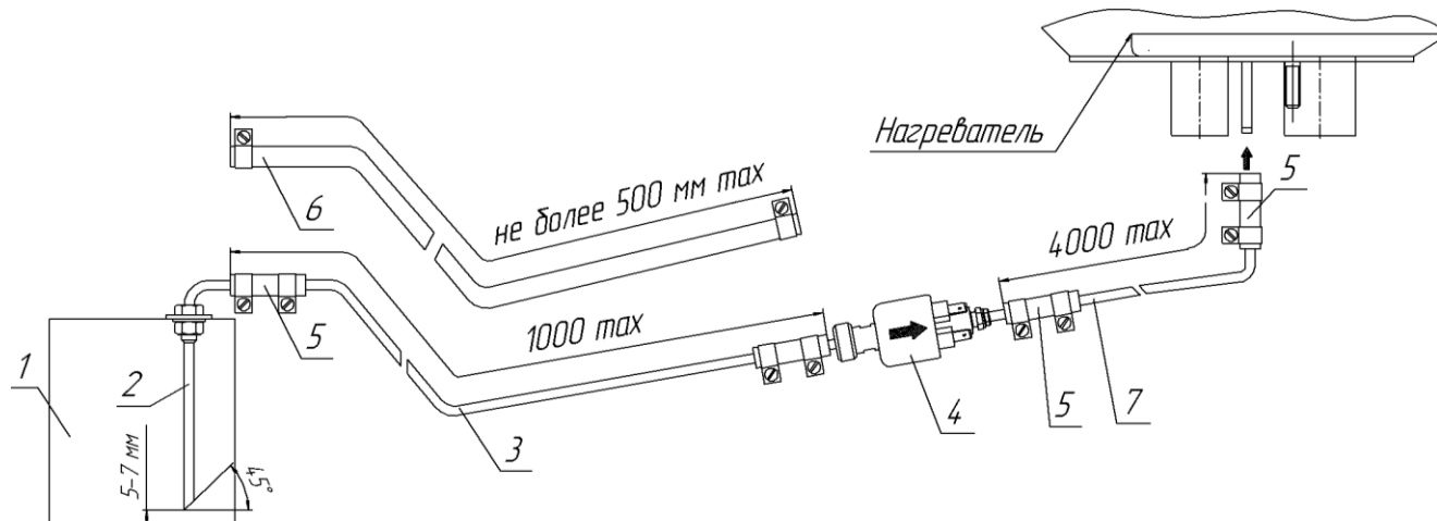
Рис. 8.5 – Монтаж топливозаборника.
