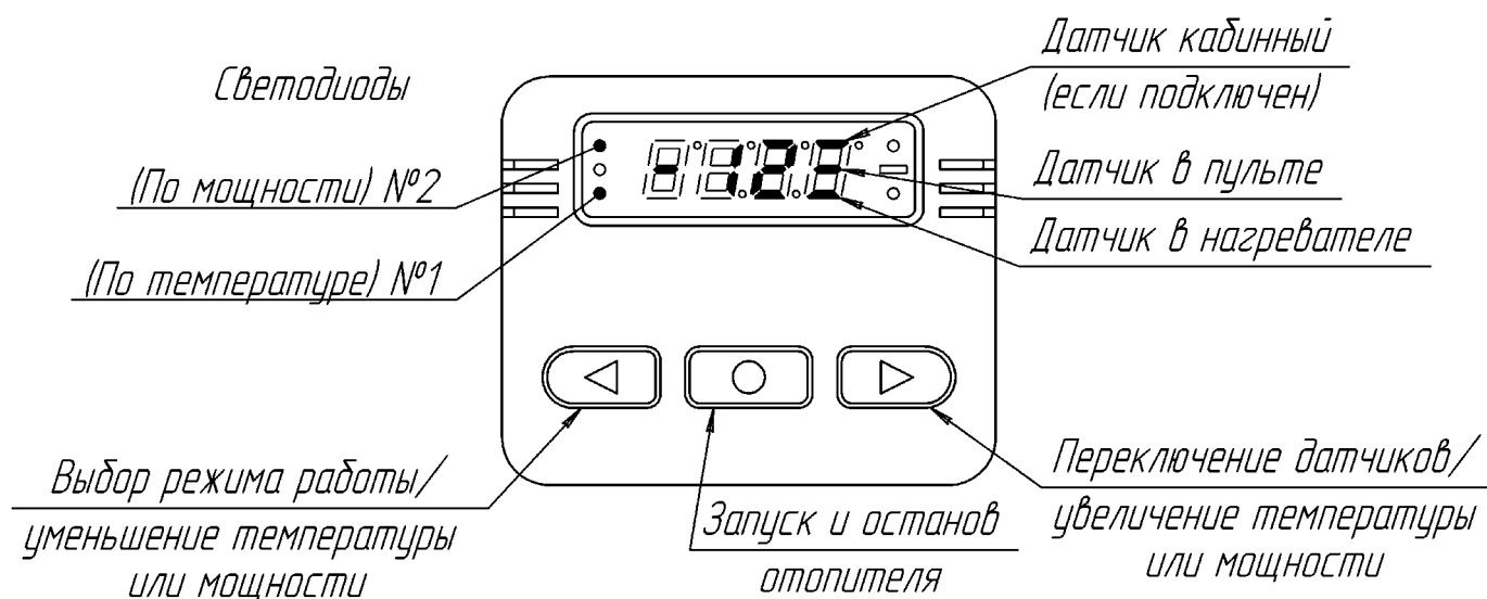
Рис. 6.2.1- Панель пульта
