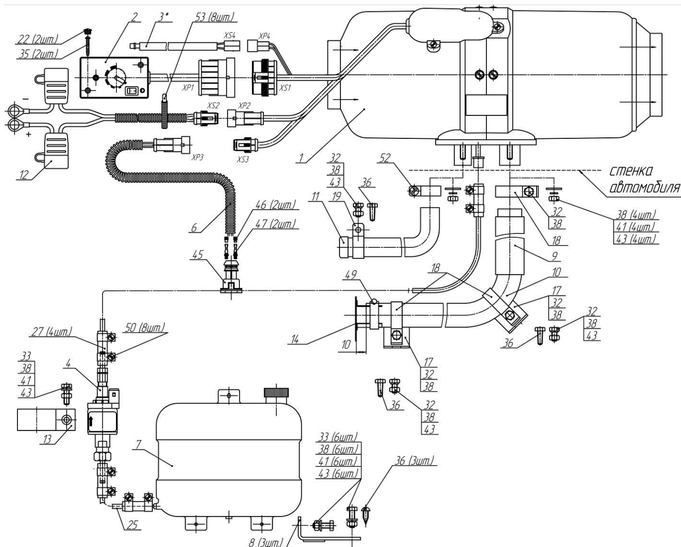
7.1 – Схема соединений основных узлов и деталей отопителя
