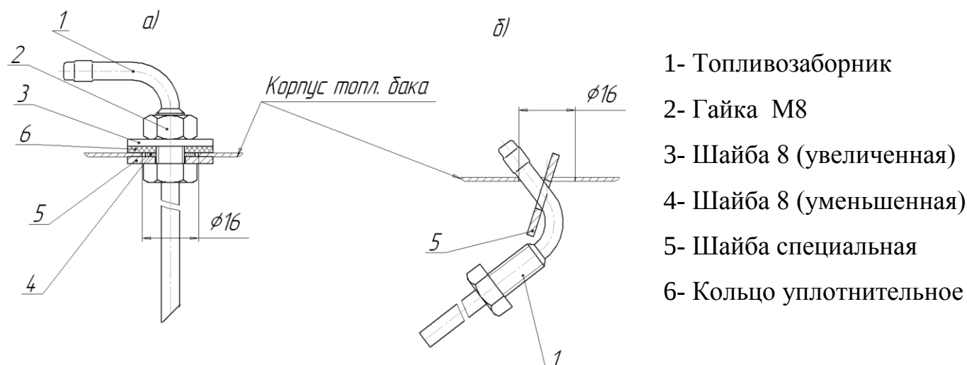
Рис. 8.4 – Монтаж топливозаборника.
